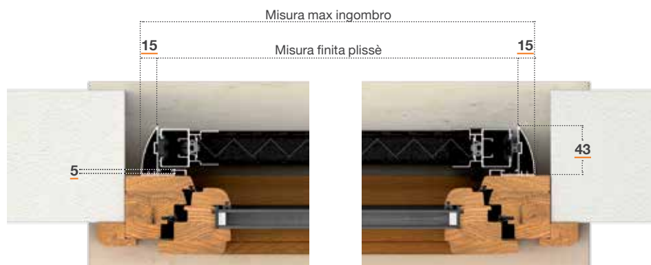
SEZ. ORIZZONTALE
