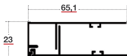
GUIDA CON TELAIO RINFORZATO
