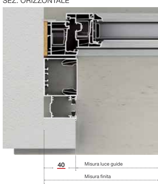
SEZ. ORIZZONTALE
