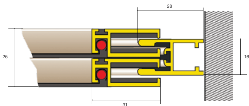
SEZ. ORIZZONTALE PANNELLI SCORREVOLI
