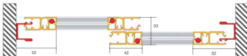
SEZ. ORIZZONTALE
