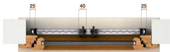
SEZ. ORIZZONTALE 2 ANTE
