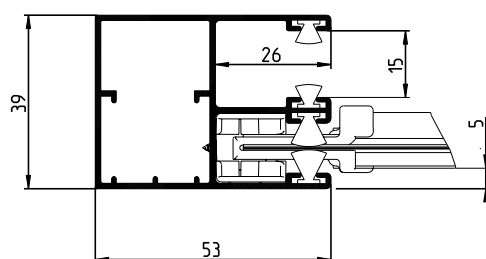
SEZIONE GUIDA
