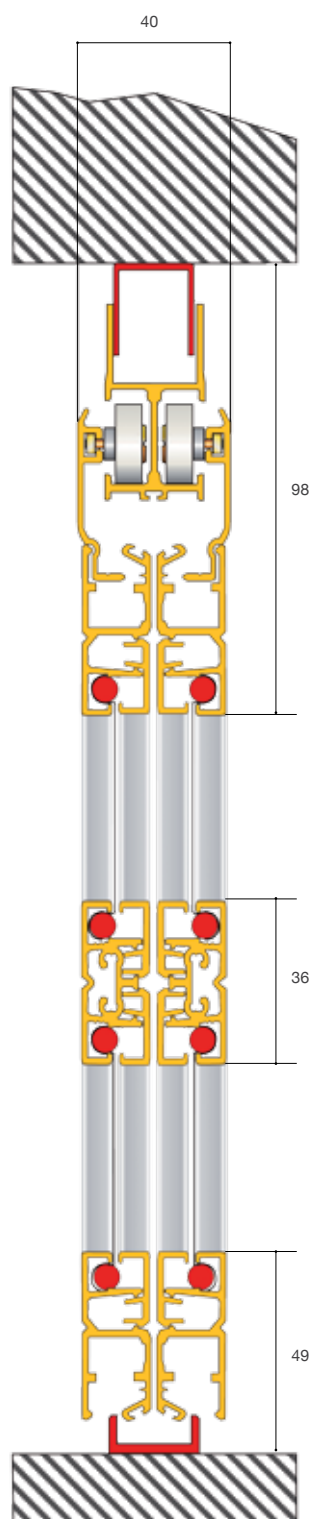
SEZ. VERTICALE
