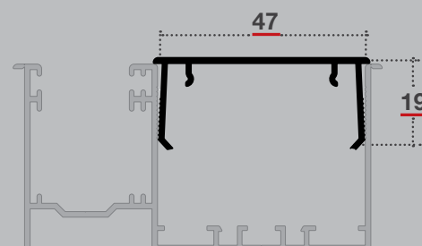
CARTER IN ALLUMINIO INCASSATA 45
