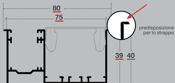
PROFILO INCASSATA 45
